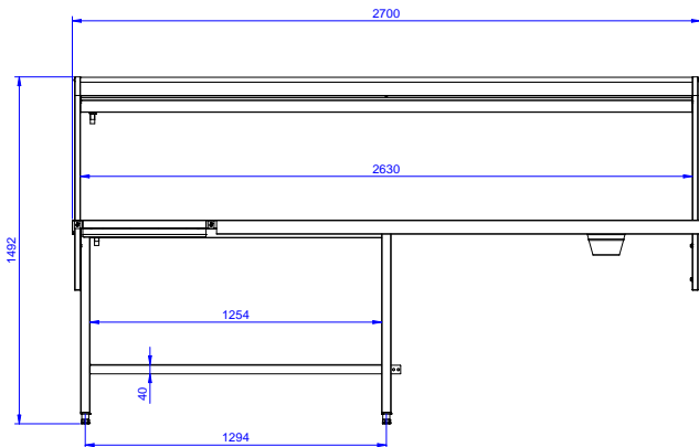
Fronte
